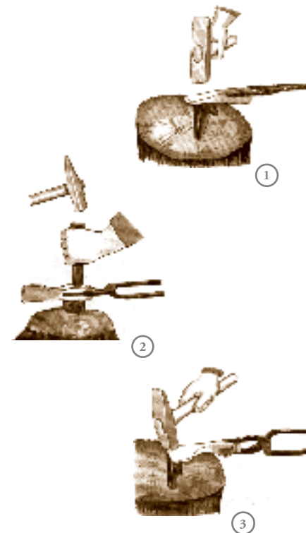
Illustrationen von N.N. Eremina-Enander aus dem Buch „Klassiskt Järnsnide“. Darin dokumentiert der Schmied L. Enander, wie historische Axtmodelle geschmiedet werden.
