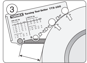
Lage der Universalstütze. Benutzen Sie Loch A oder Loch B.
