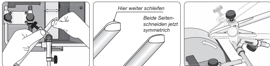
Die andere Seite in gleicher Weise schleifen. Die Gesamtbreite des Steines ausnützen. Die Form oft kontrollieren und weiterschleifen wo es notwendig ist. Den Schleifdruck reduzieren, wenn Sie die gewünschte Form erhalten haben, und das Schleifen mit einer schwingenden Bewegung des Drehrohrs beenden.
