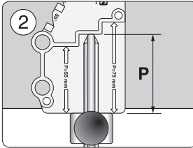
Überstand des Werkzeugs, P.
